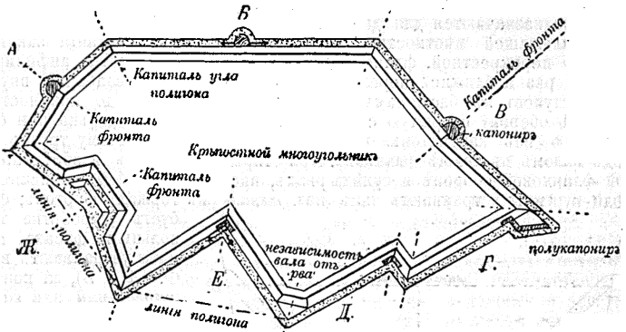
Черт. 1. А, В, С, Г—полигональные фронты; Д—кремльберный; Е—тенальный, Ж—бастіонный.
